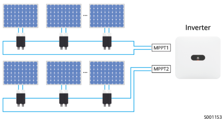
Abbildung 2-2 Anwendungsszenario (Optimierer für alle an einen Wechselrichter angeschlossenen PV-Module konfiguriert)
