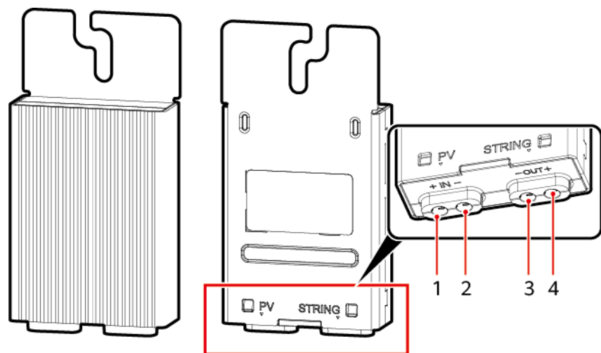
Abbildung 2-5 Anschlüsse
