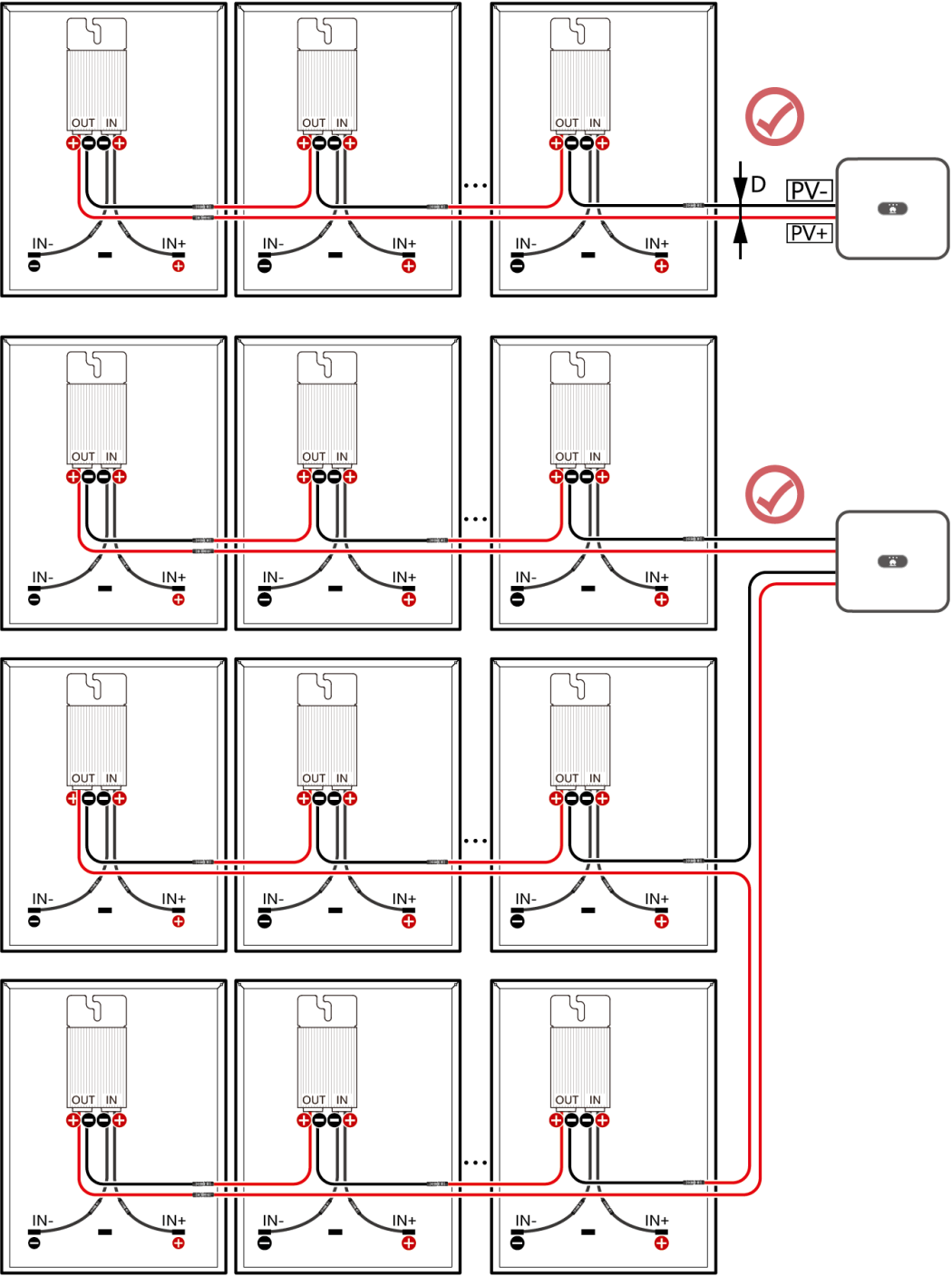
Abbildung 3-8 Erforderliche Verkabelung
