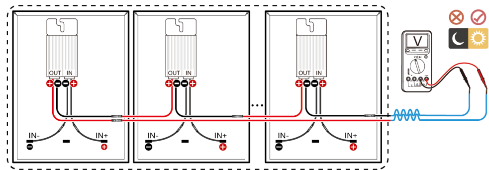
Abbildung 3-7 Messen der PV-String-Spannung
